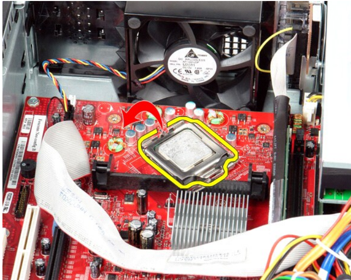
7. 컴퓨터에서 프로세서를 분리합니다.
