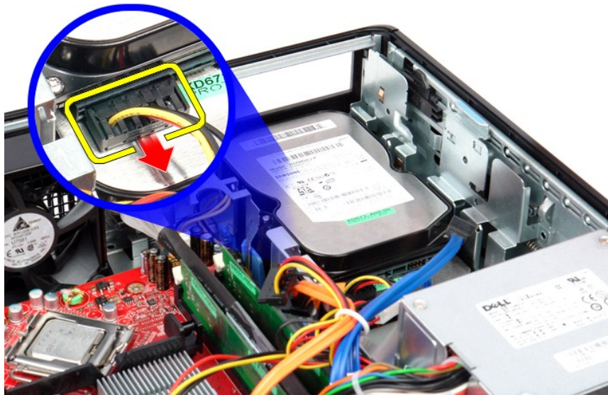
5. 분리 래치를 위로 당긴 다음 하드 드라이브를 컴퓨터 후면으로 밀습니다.
