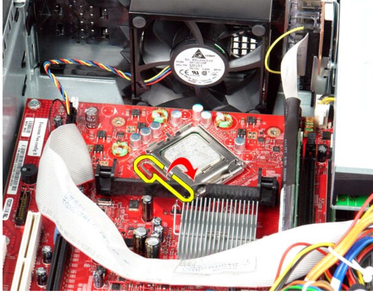
6. 프로세서 덮개를 들어 올립니다.
