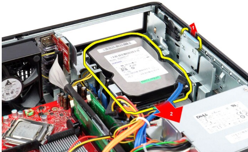
6. 하드 드라이브를 들어 올려 컴퓨터에서 분리합니다.
